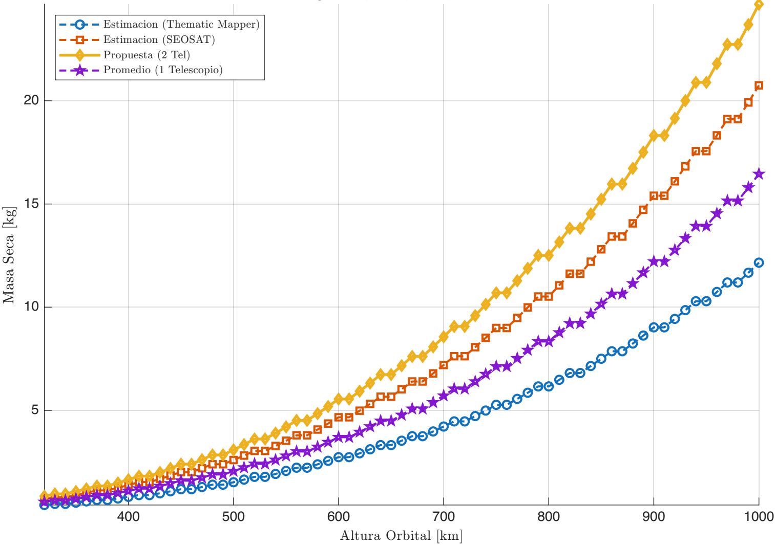
Comparativa de Masa Seca vs. Altura Config: 1 Sat, 2 Tel, Det 1, Refractivo
